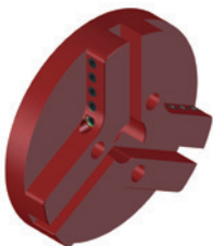
Set za proširenje za OD Ø do 140 mm (5.51") uključujući 140 mm disk vretena i blokovi čeljusti (7, 8, 9) – 3 seta Šifra proizvoda: ZST-0472-15-00-00-0
